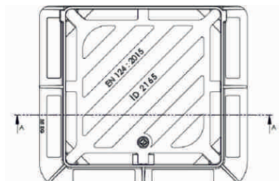
Capace și grătare din fontă sau neopren
